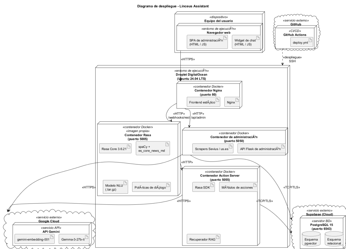
Figura 7.2: Diagrama de despliegue del sistema Linceus en DigitalOcean (Ubuntu 24.04 LTS) con el pipeline de despliegue automatizado vía GitHub Actions.
